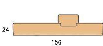
在来用固定枠
