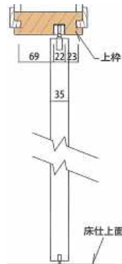
鴨居シングル
