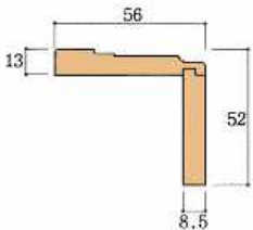
WDC-42-7 or 12 H3004額縁付延長
