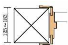
WDC-42-7 or 12 H3004額縁付延長
