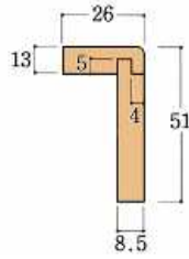
平額縁付延長
