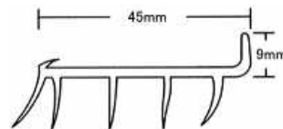
ドアボトムス (ボトムウェザーストリップ)
